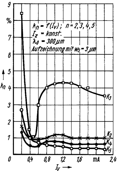
Bild 9.9. Klirrkoeffizienten in Abhängigkeit vom Vormagnetisierungsstrom
